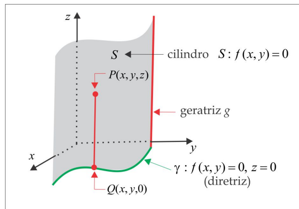
Figura 4.2: Cilindro Reto.
