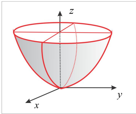
Figura 4.7: Paraboloide de Revolução
