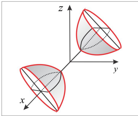
Figura 4.9: Hiperboloide de duas Folhas
