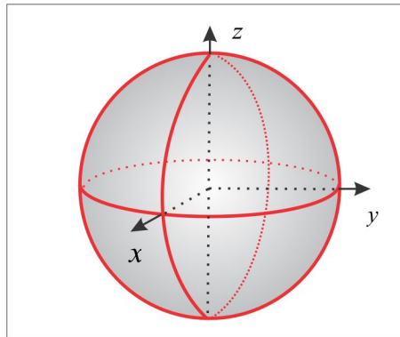
Figura 4.6: Esfera.
