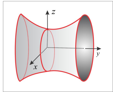
Figura 4.10: Hiperboloide de uma Folha
