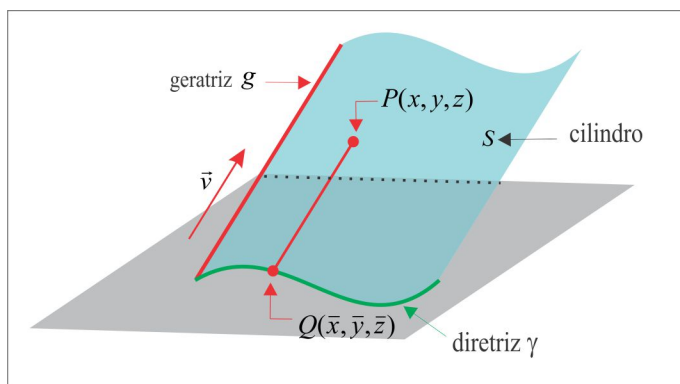
Figura 4.1: Superfície Cilíndrica.
