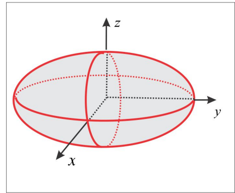
Figura 4.8: Elipsoide de Revolução
