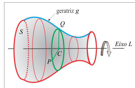
Figura 4.5: Superfície de Revolução
